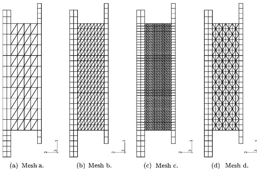
Fig. 9. Mesh refinement.
